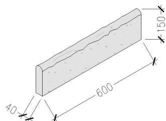
Old Town obrubník 60/4/15 cm
