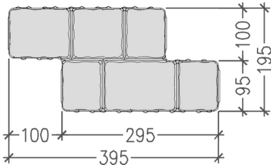
Typ „A“ - 40 x 20 x 8 cm
